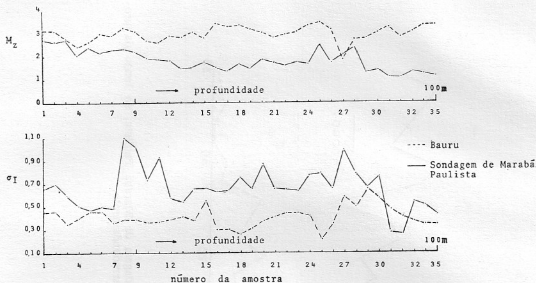
Fig. 3 — Variação do Tamanho Médio ( M_z ) e do Desvio Padrão ( \delta I ), com a profundidade, de sedimentos do Bauru e da sondagem de Marabá Paulista. O Bauru se mostra mais fino e melhor selecionado que as amostras da referida sondagem.
