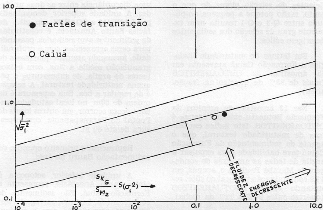
Fig. 5 — Diagrama de Sahu aplicado ao sedimento da sondagem de Marabá Paulista, sugerindo ambiente deltaico de deposição para a fácies de transição e para o Caiuá.
