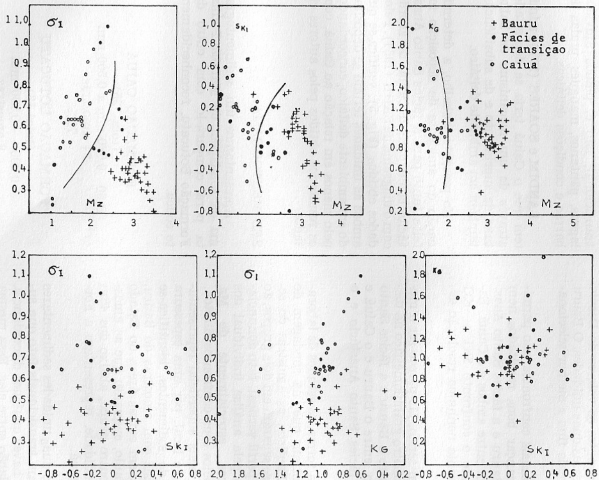
Fig. 4 — Confronto de parâmetros granulométricos de amostras do Bauru, da fácies transicional e do Caiuá. Nos confrontos M_z x \sigma_1 , M_z x SK_I , M_z x KG ocorre boa resolução mostrando vinculação entre o Bauru e a Fácies de transição. Verifica-se também uma transição entre esta última e o Caiuá.
