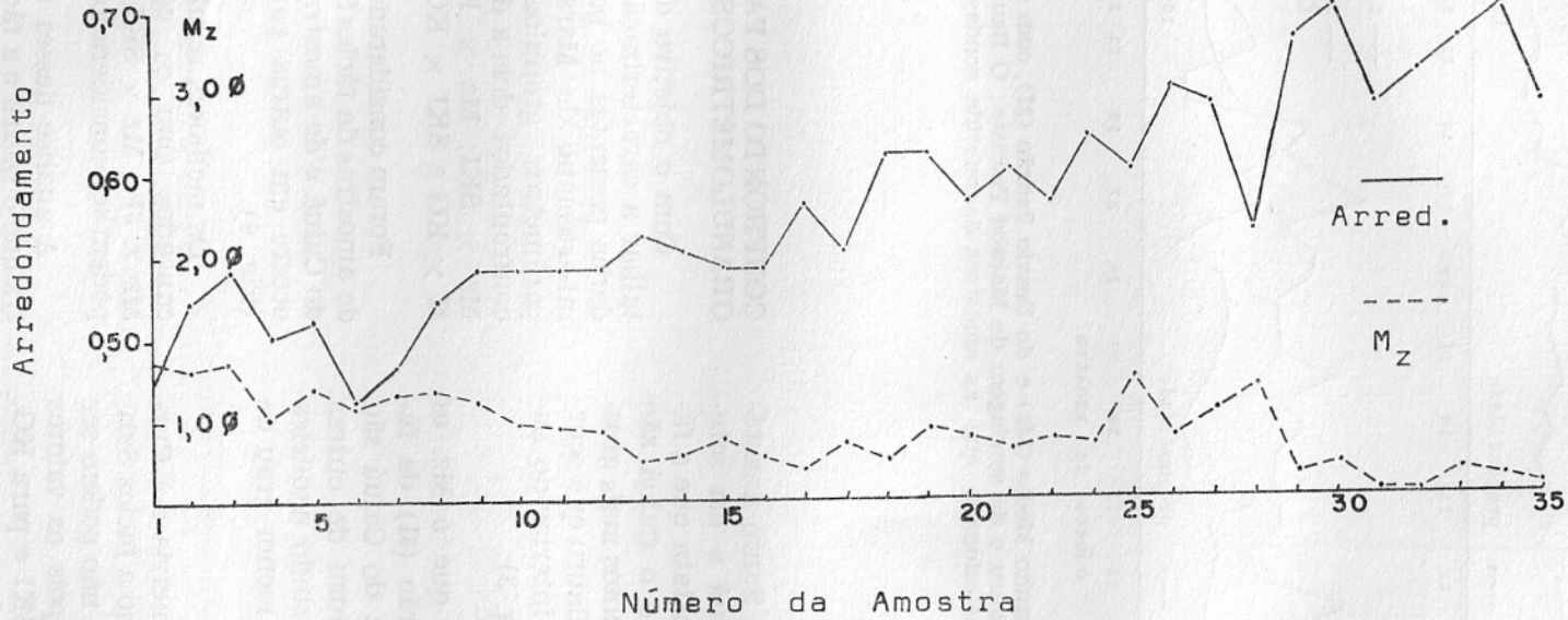
Fig. 2 — Variação do arredondamento e do Tamanho Médio (Mz) do sedimento da sondagem de Marabá Paulista, ao longo da profundidade. A medida que o sedimento se torna mais grosso, maior é o seu arredondamento.
