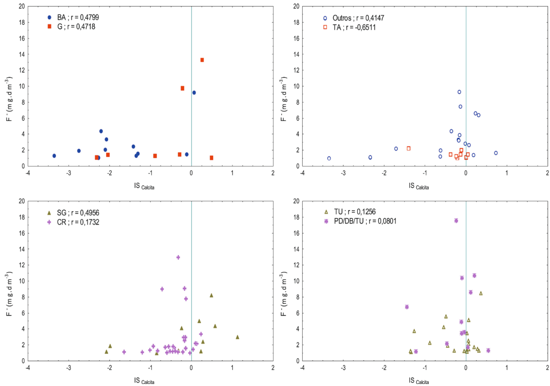
FIGURA 9 – Diagrama de Índice de saturação em calcita em relação a [F - ] (BA=Bauru; G=Guarani; SG=Serra Geral; CR=Cristalino; TA=Taubaté; Outros= Diabásio, poços mistos; PD =Aquitarde Passa Dois; TU=Tubarão).
