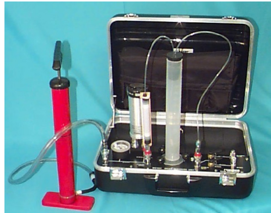
FIGURA 7 – Acessório da Pylon para determinação de ^{222}\text{Rn} dissolvido em água (Radioactive Products | Pylon Electronics-Radon ( pyronelectronics-radon.com )).
